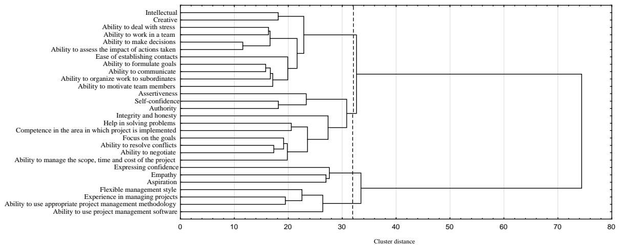
Fig. 2. Dendrogram.
